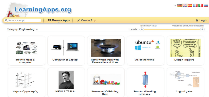
Рис. 2. Web-сервіс LearningApps.org
