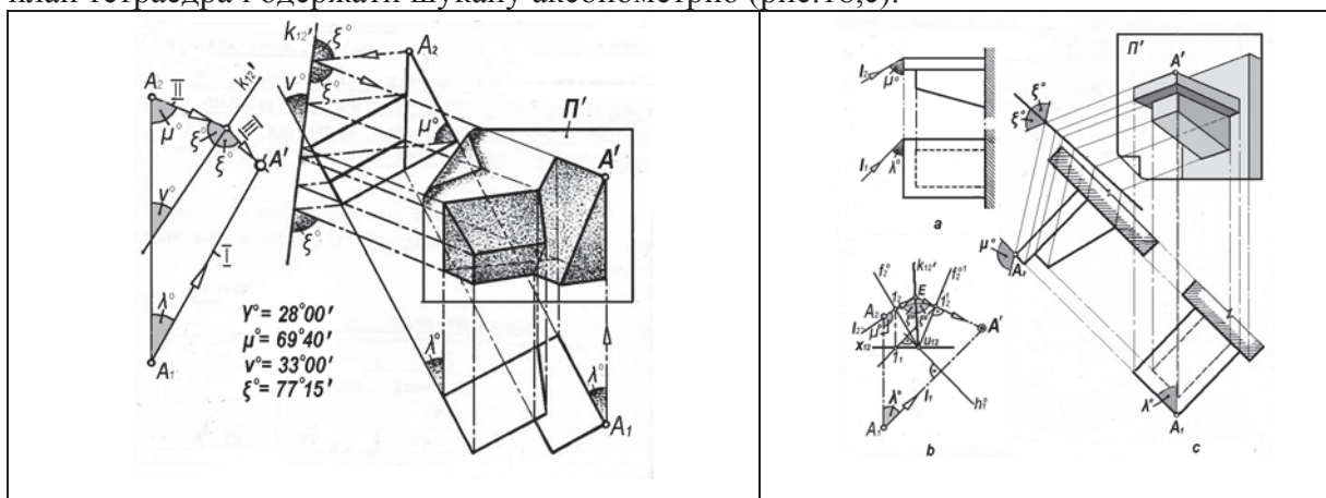
Рис. 19. Приклад побудови точної триметрії об'єкта методом параметрів аксонометричного проєціювання
