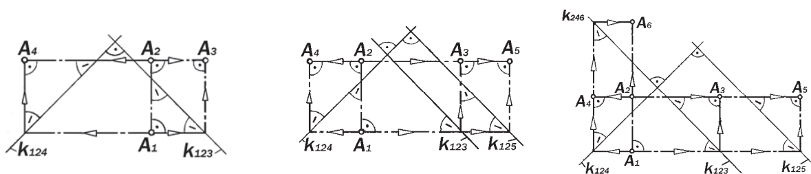
Рис. 2. Геометрична модель апарату одержання багатокартинних комплексних креслень
